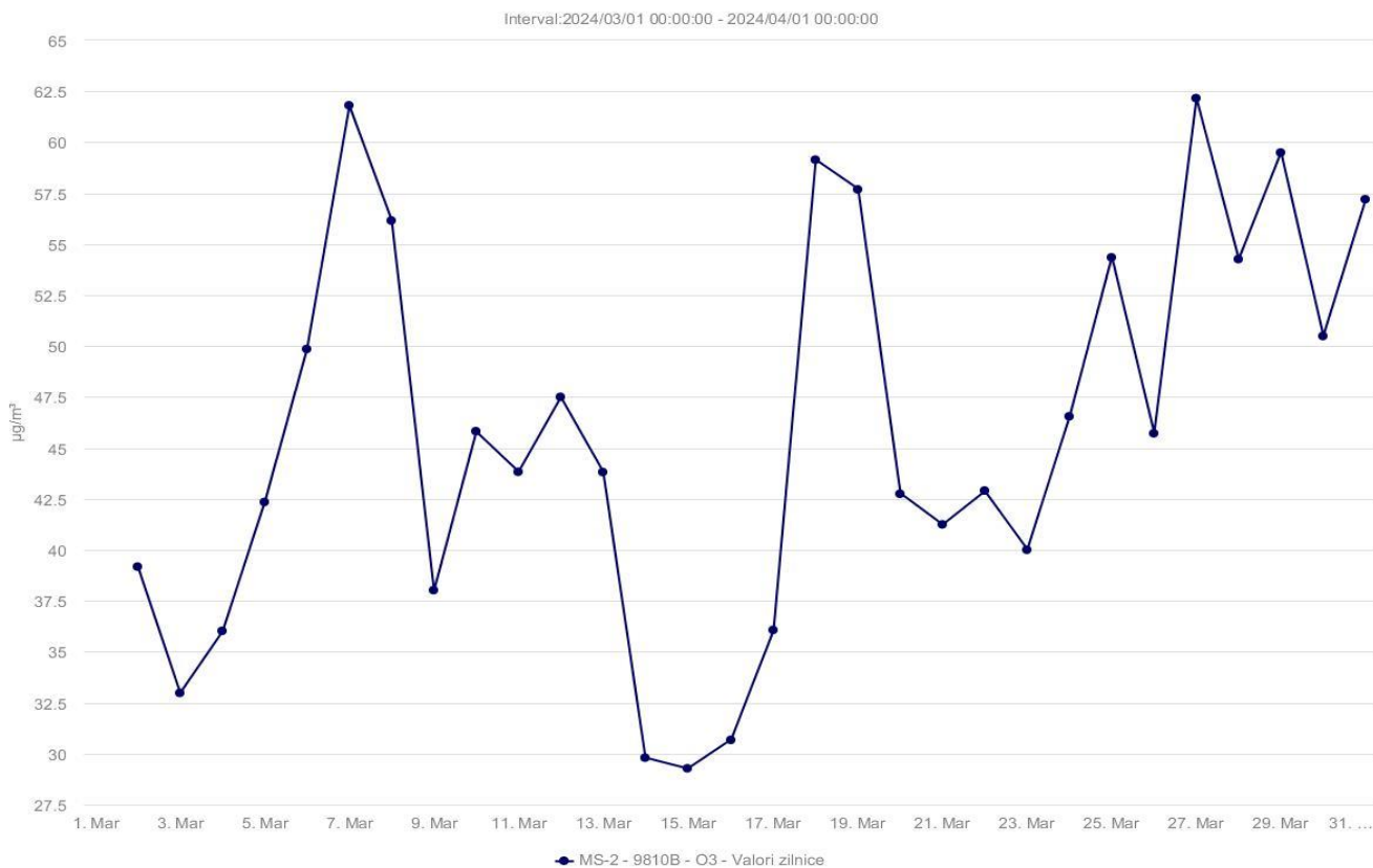
Evoluția valorilor medii zilnice ale indicatorului ozon (O 3 ) la stația MS-2
