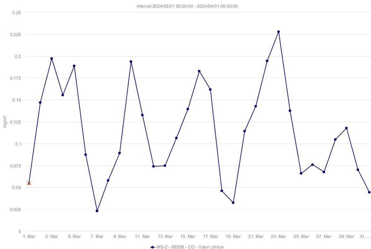
Evoluția valorilor medii zilnice ale indicatorului monoxid de carbon (CO) la stația MS-2
