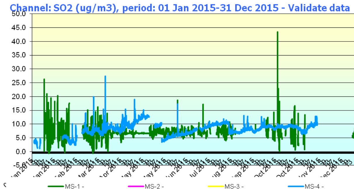
Varianța concentrației dioxidului de sulf – medii orare
