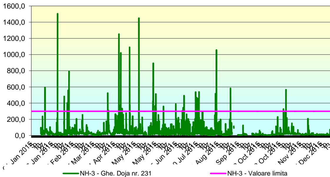
Evoluția concentrațiilor medii momentane pentru amoniac - NH 3 (ug/m 3 ) - anul 2015
