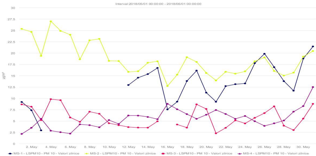
Evoluția valorilor medii zilnice ale indicatorului Pulveri in suspensie fracția PM 10 la stațiile de monitorizare din județul Mureș
