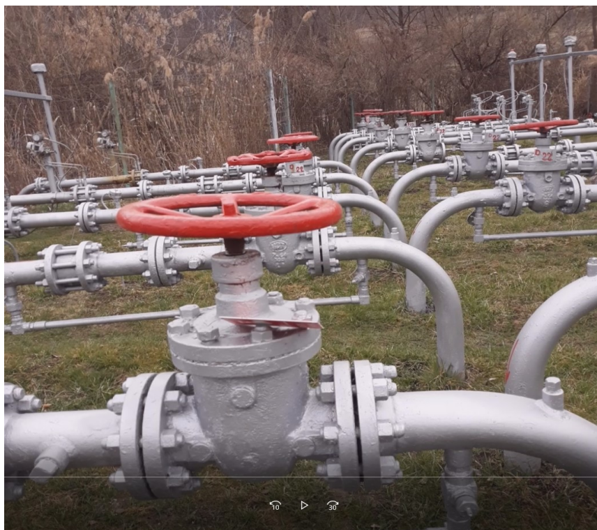
Zona de adaptare a instalatiei tehnologice in vederea montarii unui compresor de camp
